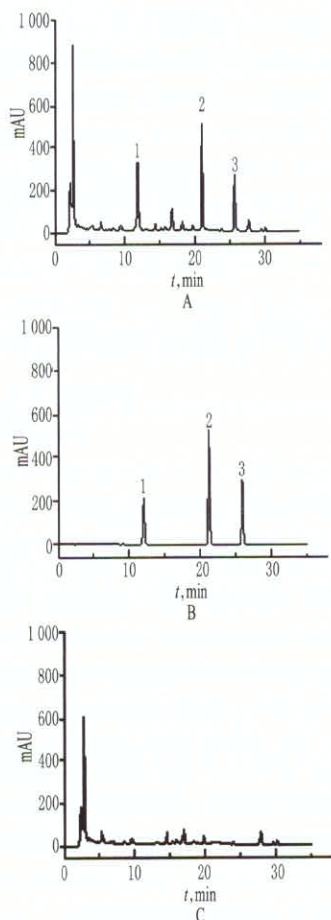
图1 高效液相色谱图
