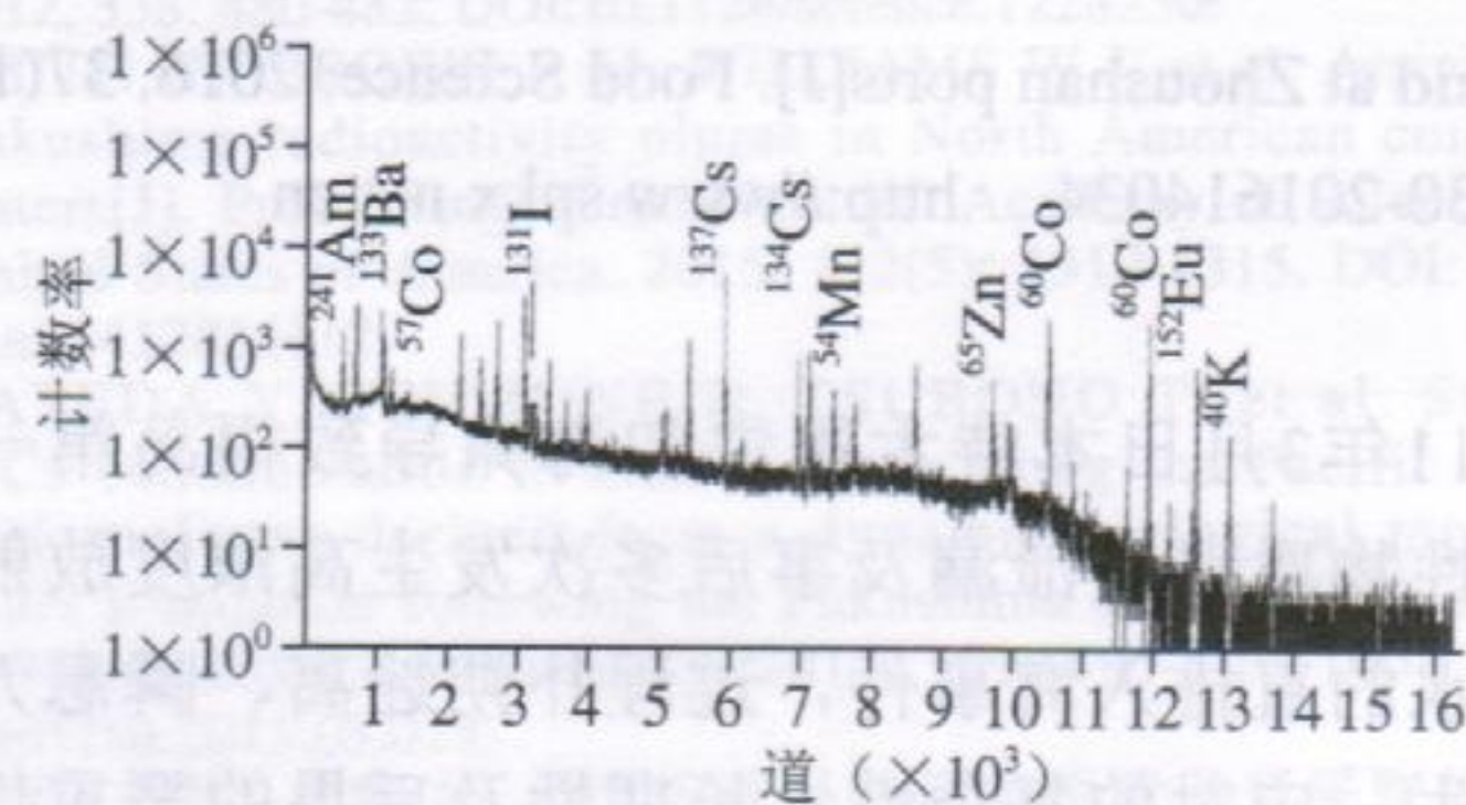
图1 生物灰标准源 \gamma 能谱图
