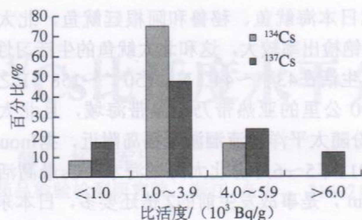
图4 阳性样品中 ^{134}\text{Cs} 和 ^{137}\text{Cs} 的比活度分布情况
