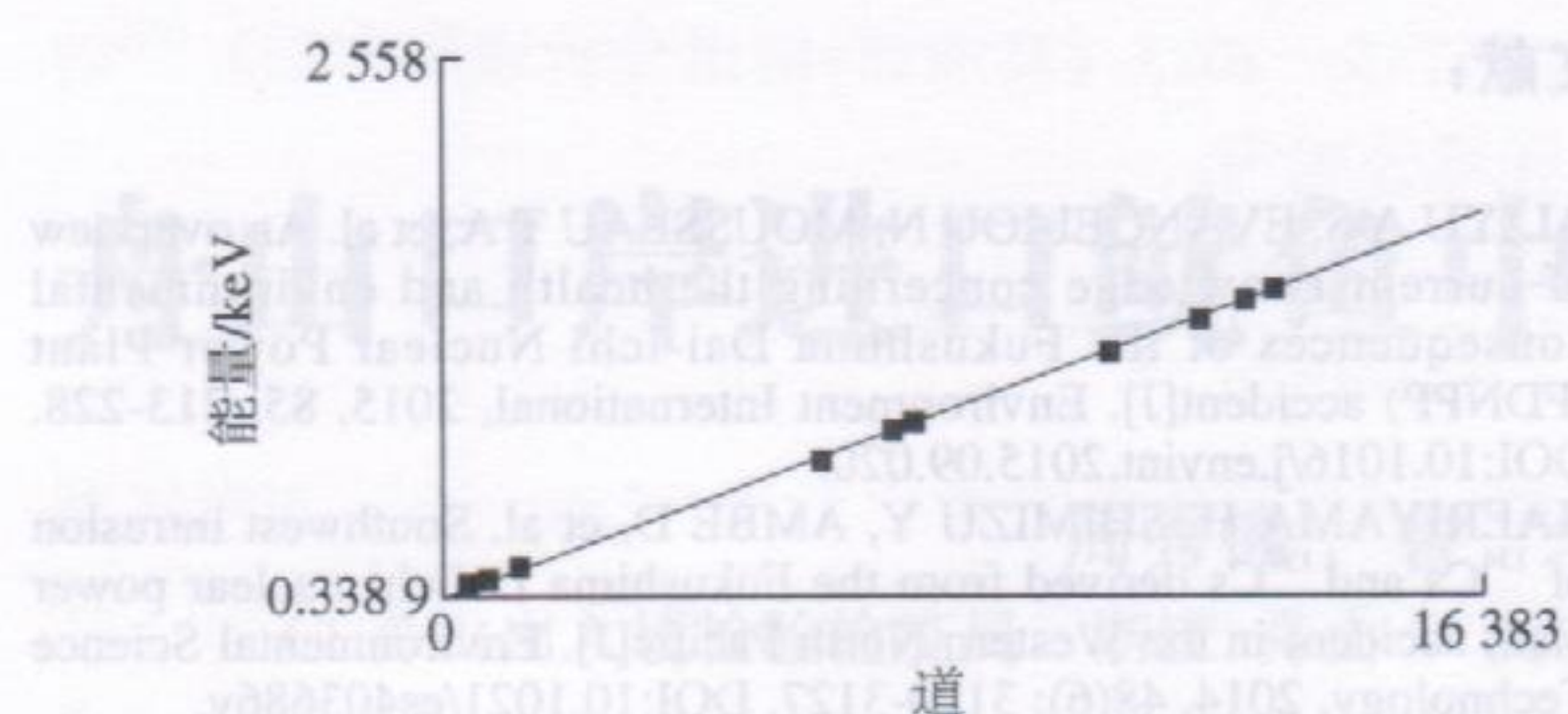
图2 放射性核素的能量刻度曲线
