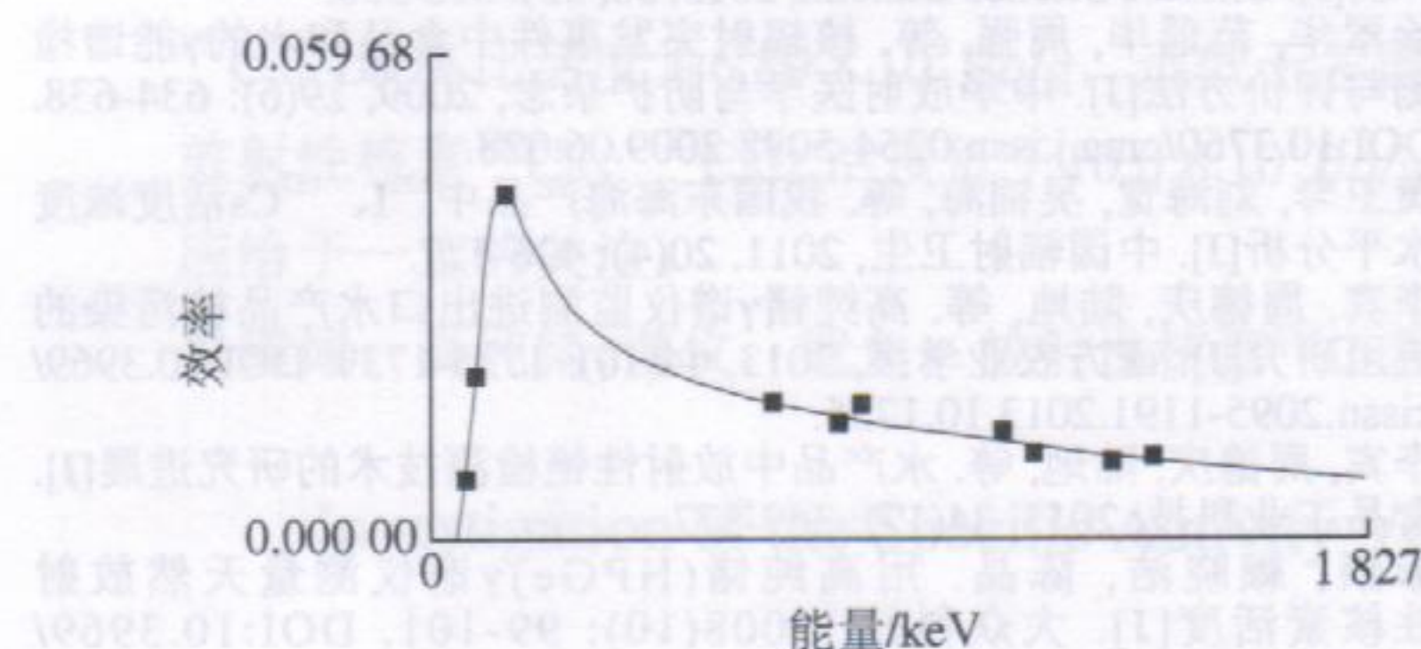
图3 放射性核素的效率刻度曲线
